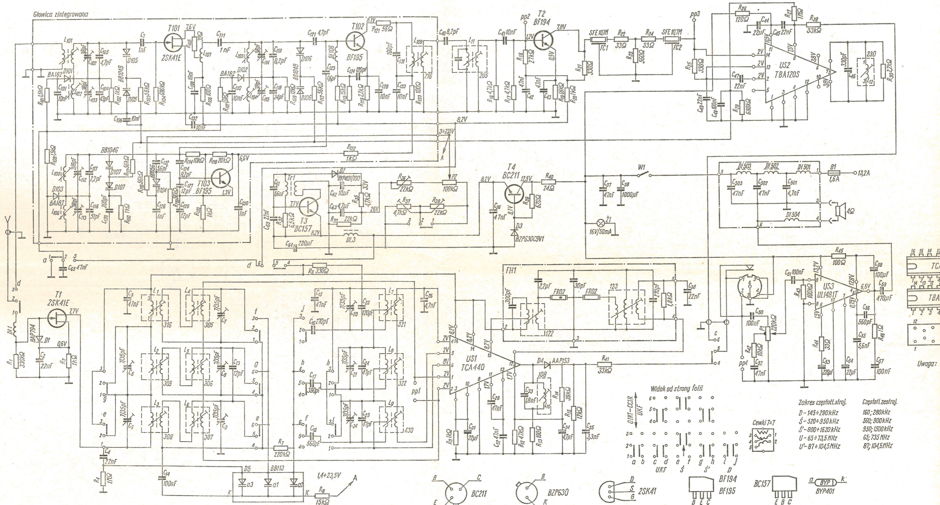
Rys. 28.35. Schemat ideowy samochodowego odbiornika radiowego „Traper” SMP-401
