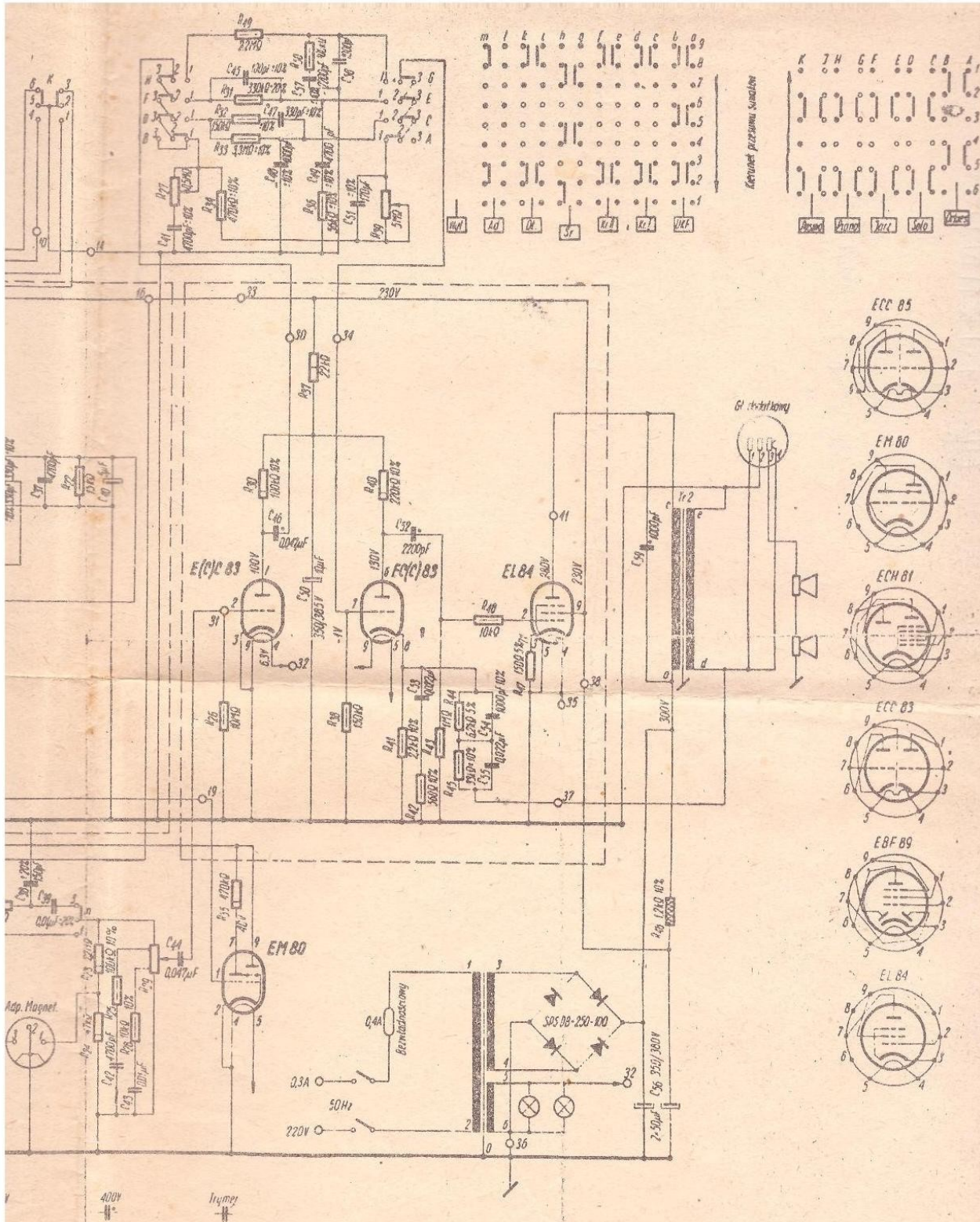
Schemat odbiornika AM/FM „Turandot“
