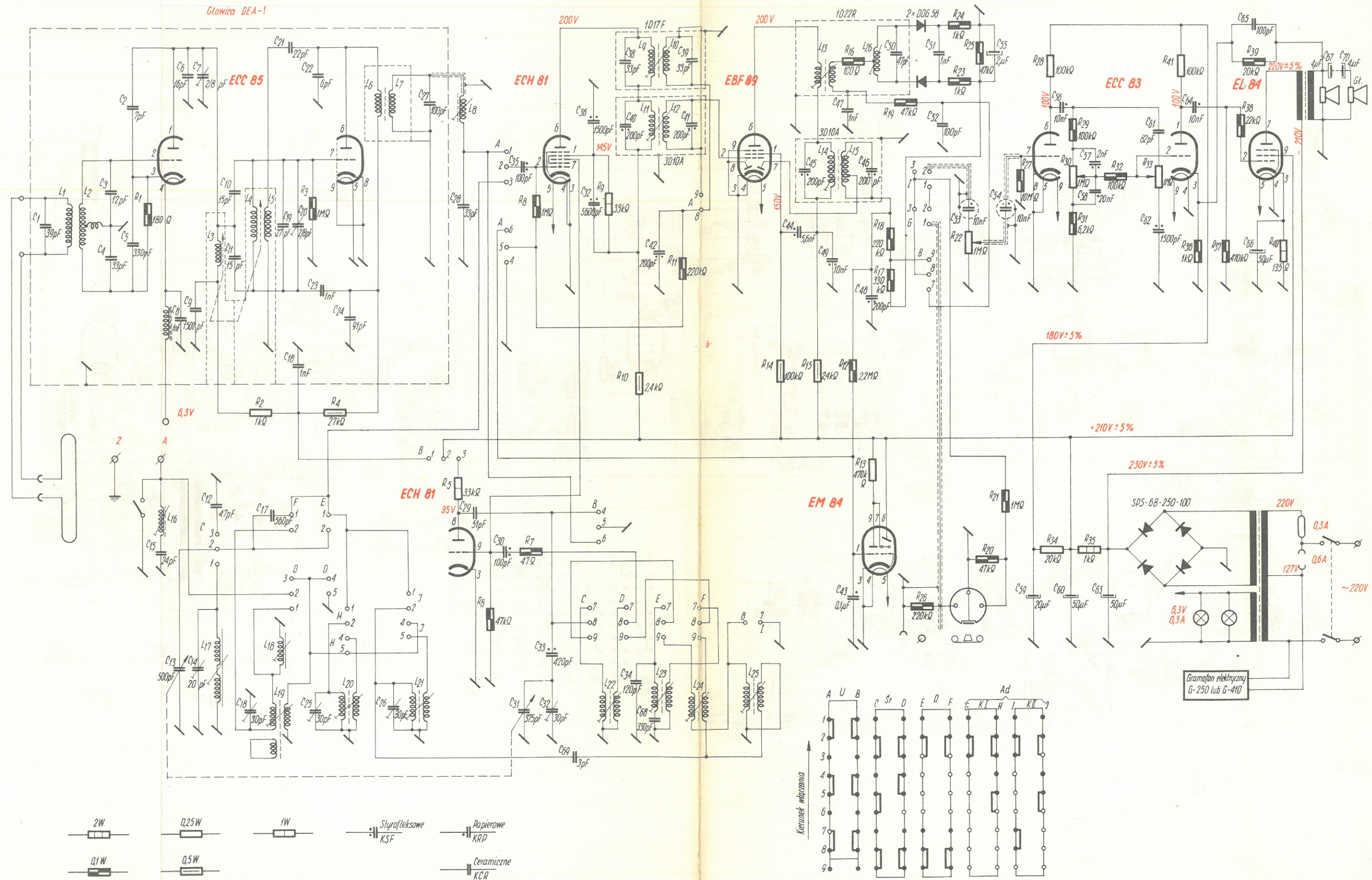
Schemat 2.10.12. Odbiornik radiowy „Aria”
