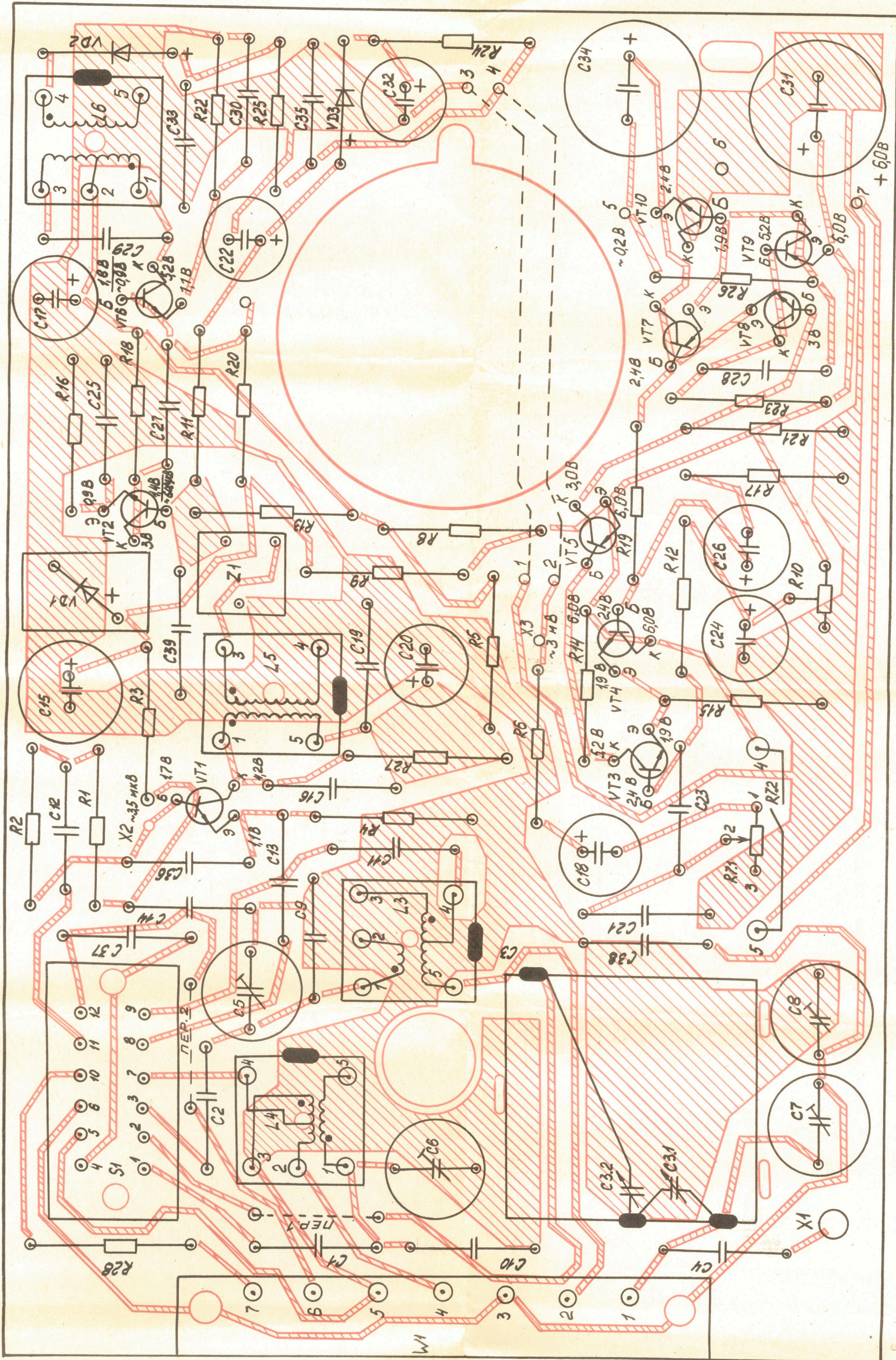
SCHEMAT MONTAŻOWY FIZYKI DRUKOWANEJ ODBIORNIKA "SOKOL-310"
